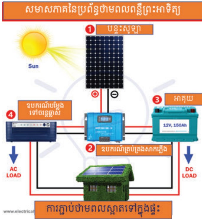
រូបភាព- ប្រព័ន្ធថាមពលពន្លឺព្រះអាទិត្យនិងសមាសភាគ
